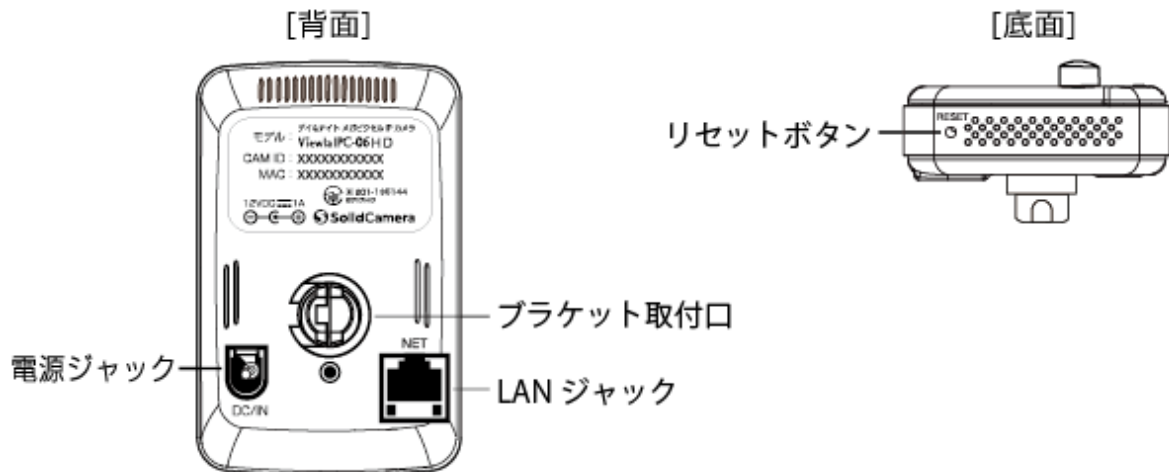
図 2-2 : 背面各部
