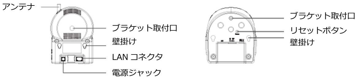
図 2-2 : 背面各部
