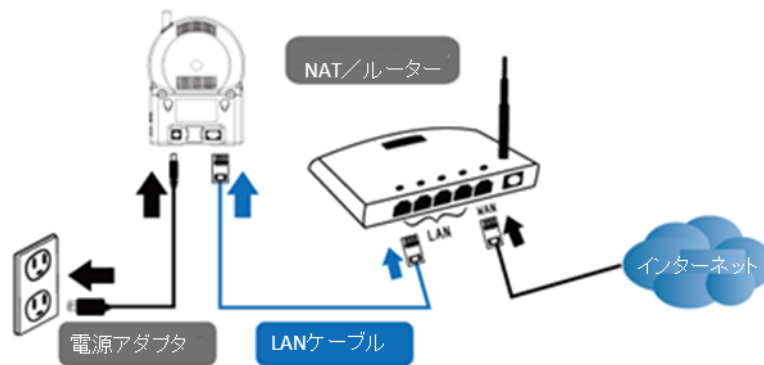
図2-9 : LAN ケーブルを抜いてWiFi 接続
