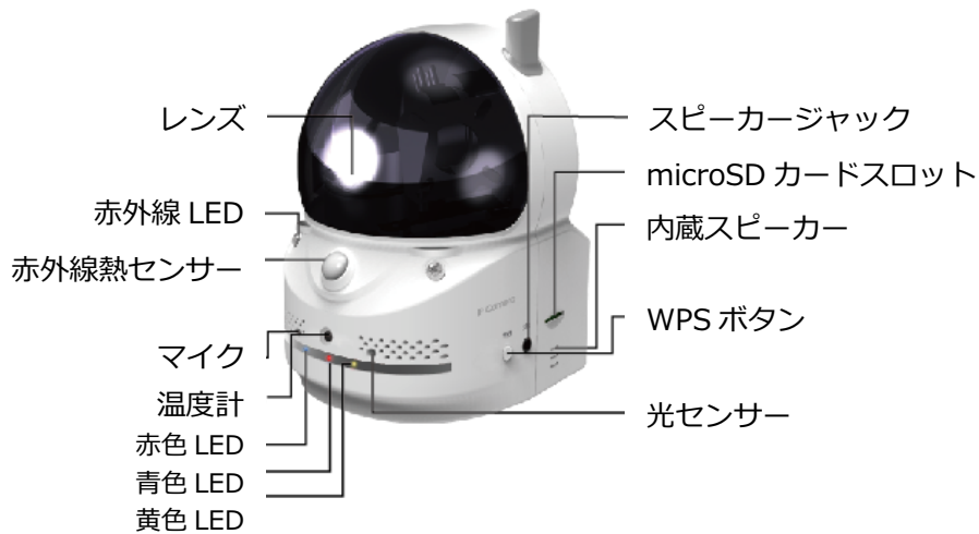
図2-1：前面・側面各部
